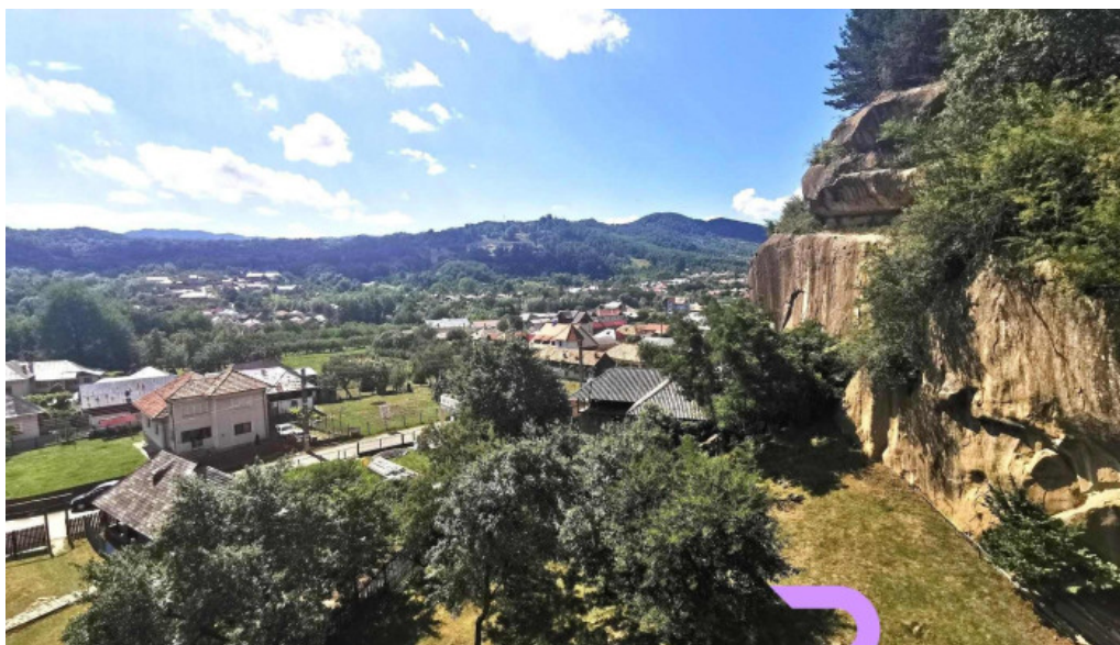
Retevoiesti scor
